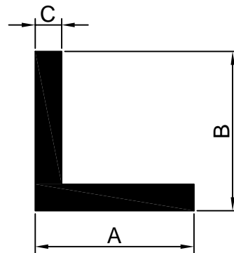
Perfil Angular
